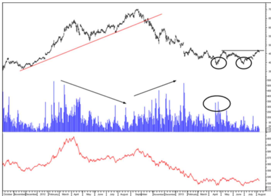
Figure 3-1: : On-balance volume.
